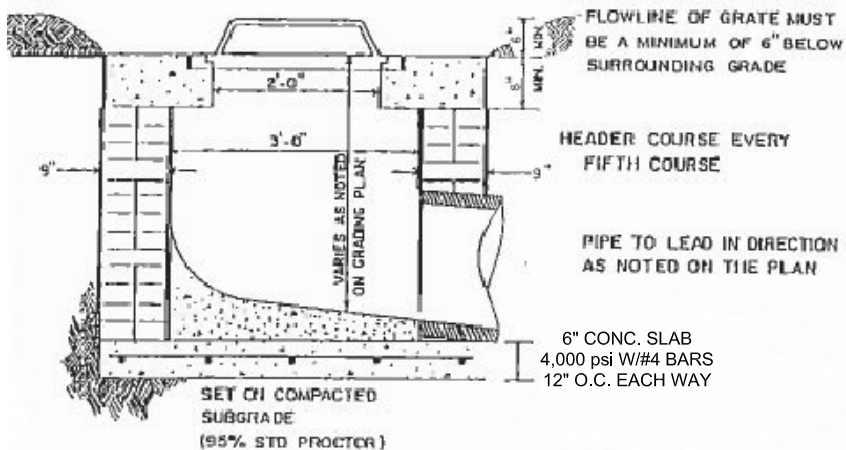
LONGITUDINAL SECTION
