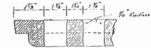
SECTION A-B
